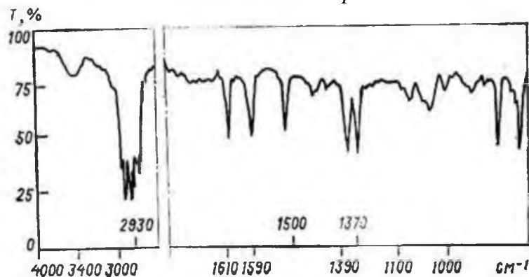
Рис.1. ИК-спектр соединения с брутто-формулой C_3H_8O .
