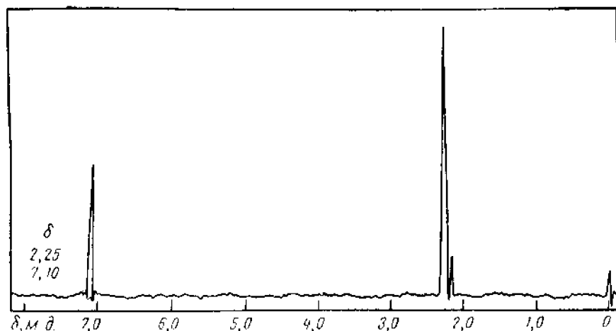
Рис. 3. ПМР спектр соединения с брутто-формулой C_8H_{10}
