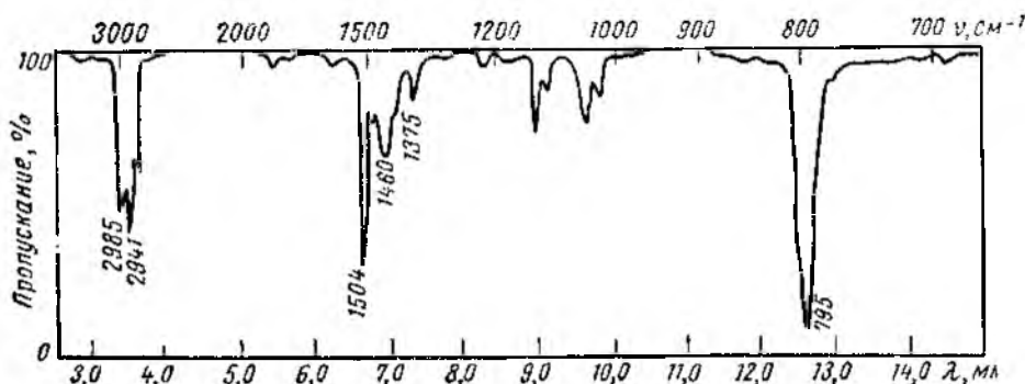
Рис. 2. ИК-спектр соединения с брутто-формулой C_8H_{10}
