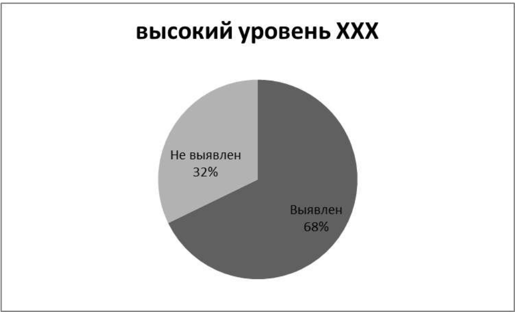
Рис.2 Количество респондентов с высоким уровнем XXXX
