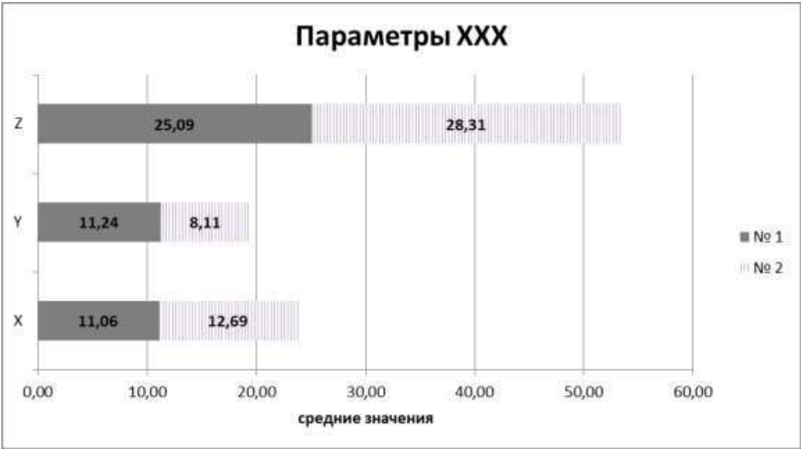
Рис.1 Распределение средних групповых значений по параметрам XXX
